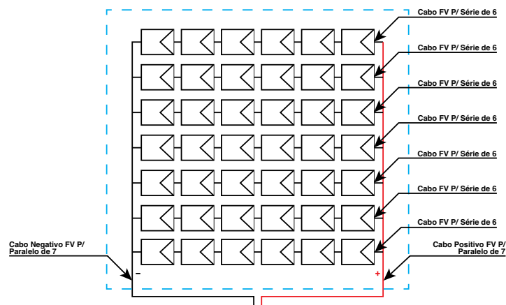
Diagrama do arranjo 6x7
