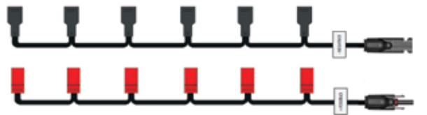
Cabeamento para o Paralelo de 6 séries
